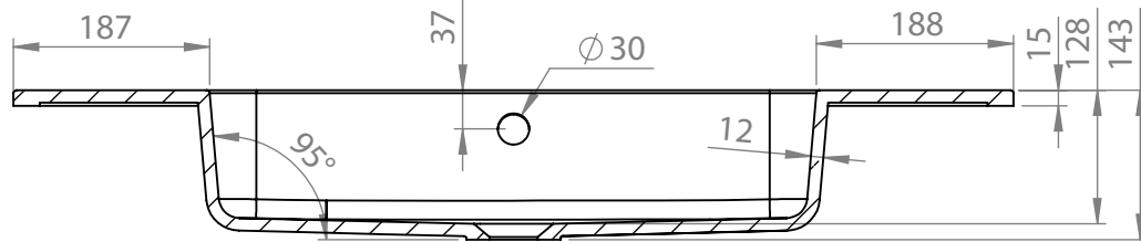
PRZEKRÓJ M-M SKALA 1 : 8
